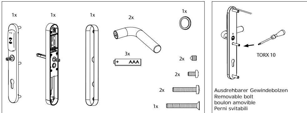
Montageanleitung / Mounting Instruction / Instructions de montage / Istruzioni di montaggio
