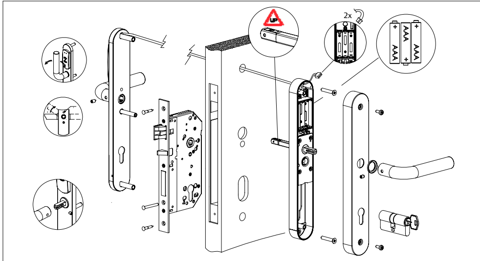
Montageanleitung / Mounting Instruction / Instructions de montage / Istruzioni di montaggio
