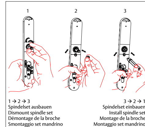
Auswechseln des Spindelsets / Spindle set replacement / Remplacement de la broche / Cambio set mandrino
